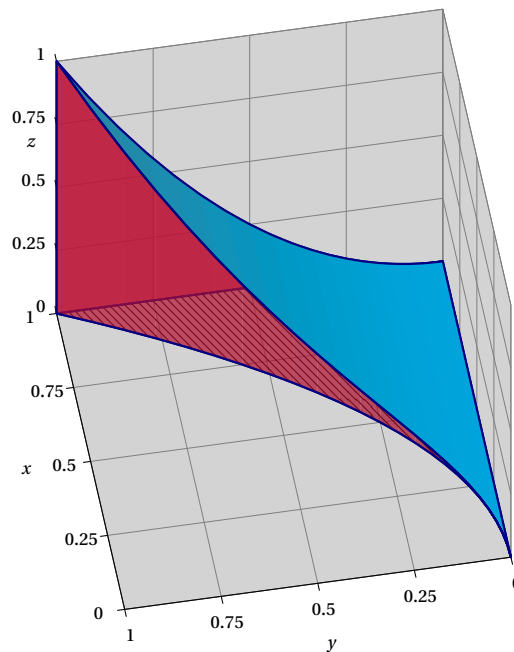
Figure 43: Volume : 0 \leq x \leq 1 ; 0 \leq y \leq x^2 ; 0 \leq z \leq y^2
